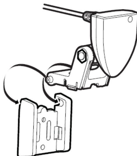
Вставка лапки пивота в кронштейн
