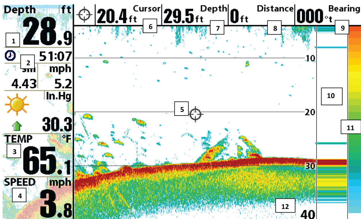
Обзор Сонара
