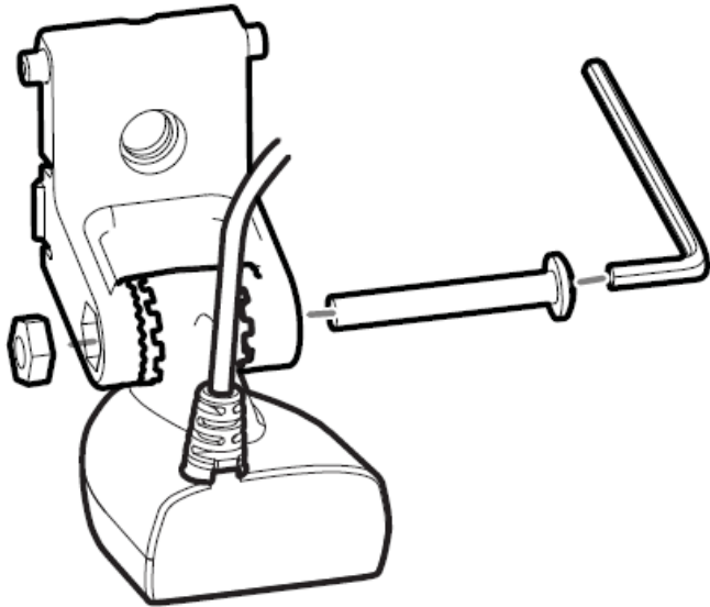
Вставка пивотного болта
