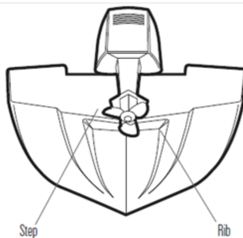
Степс - шпангоут
