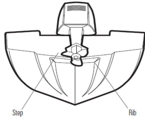
Степс - шпангоут
