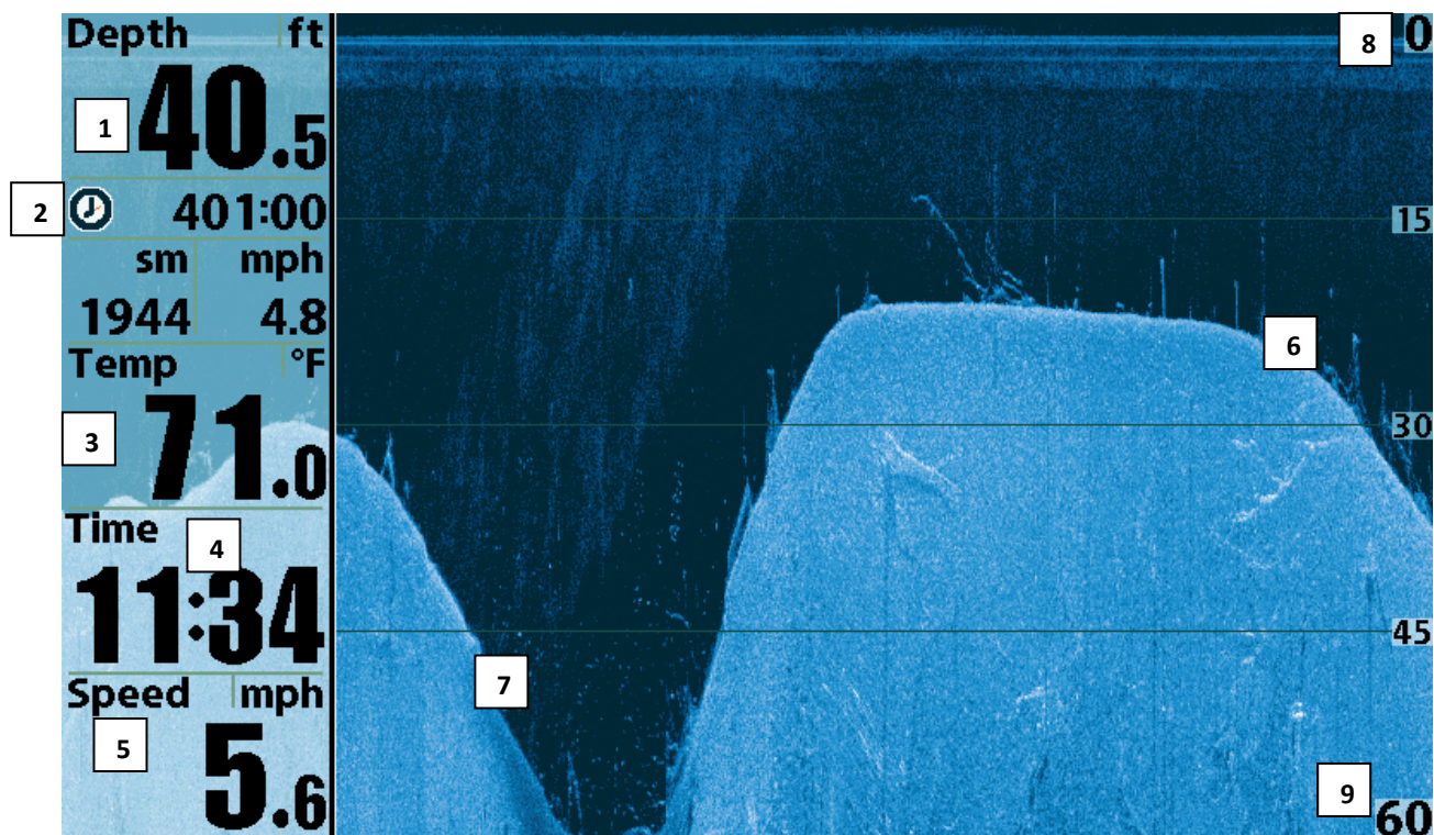
Обзор Down Imaging™
