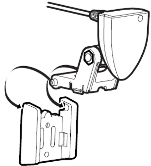
Вставка лапки пивота в кронштейн
